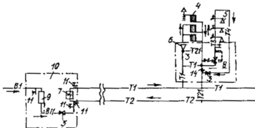
Рис. 2. Схема открытой системы теплоснабжения
