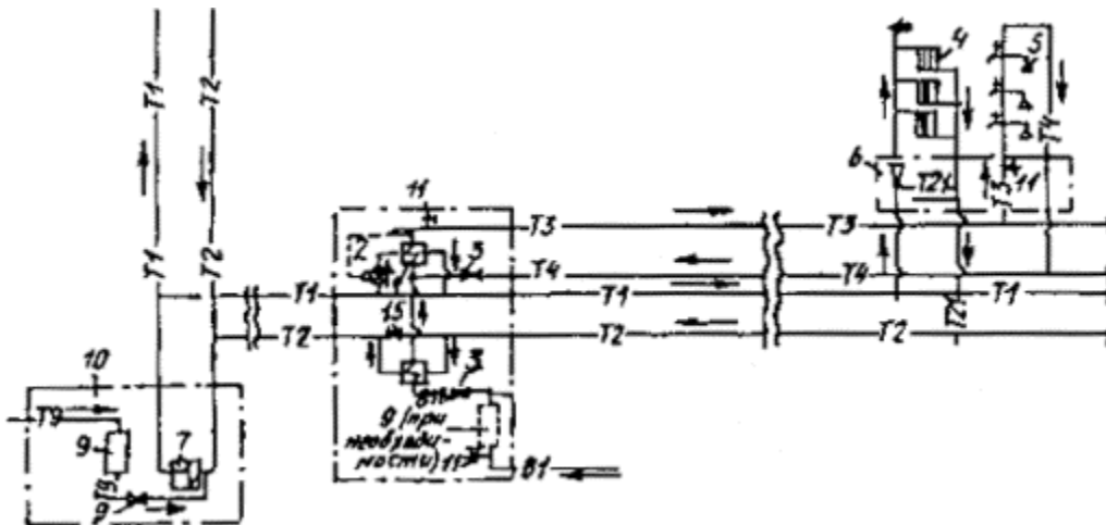
Рис. 1. Схема закрытой системы теплоснабжения
